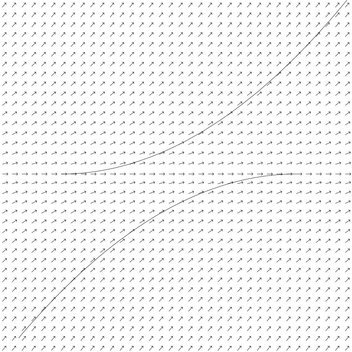
图1 微分方程式 \frac{dy}{dx} = \sqrt{|y|}
